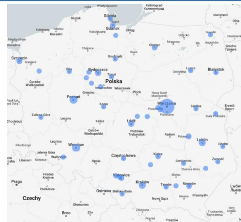
Wapnowanie gleb
